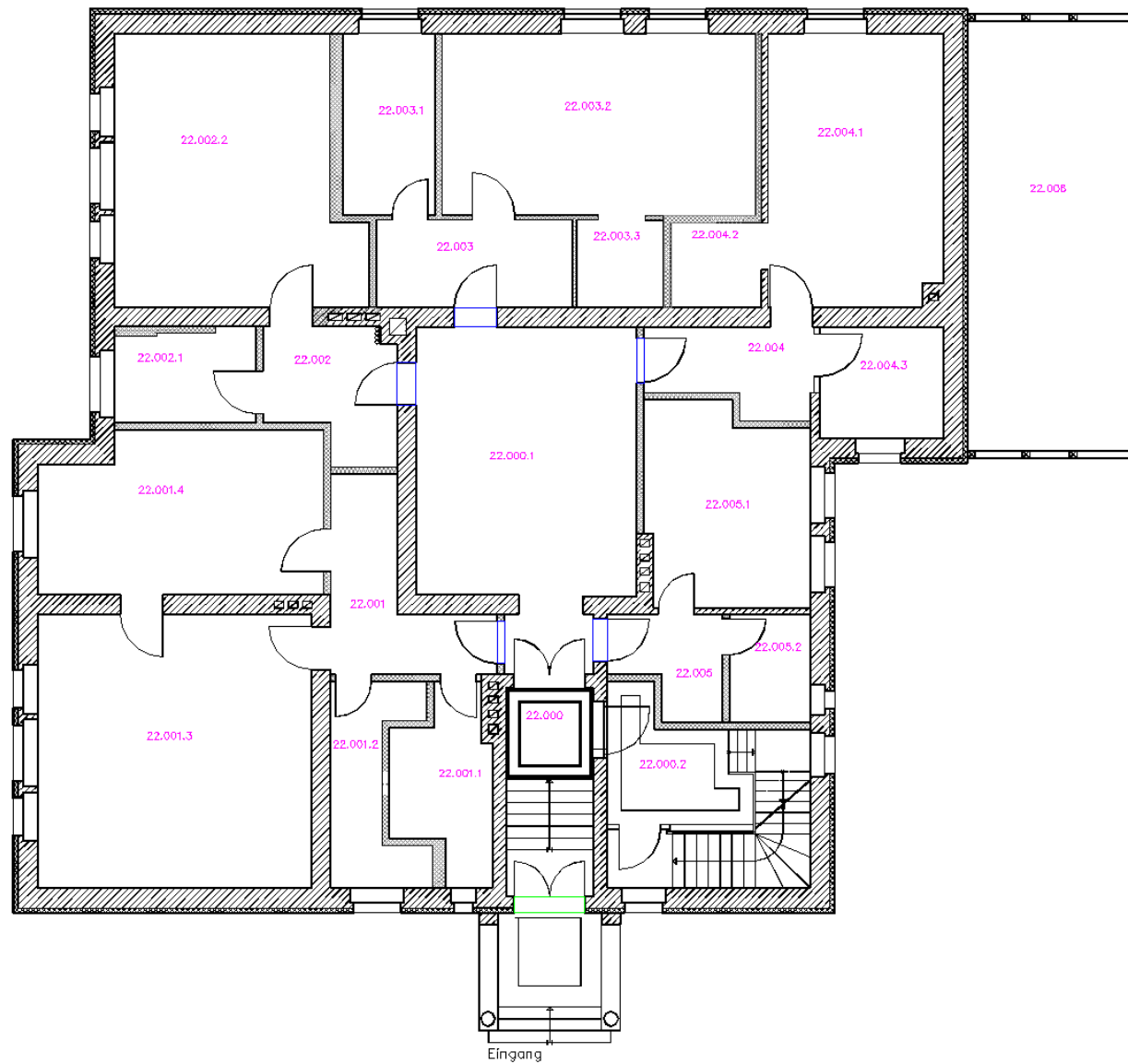
Abbildung 4: Grundriss - Erste Etage
