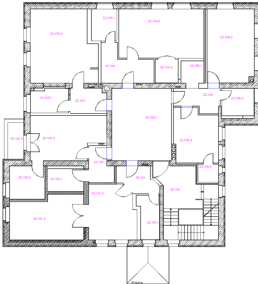
Abbildung 5: Grundriss - Zweite Etage
