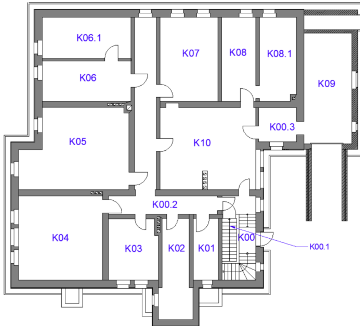
Abbildung 3: Grundriss - Kellergeschoss
