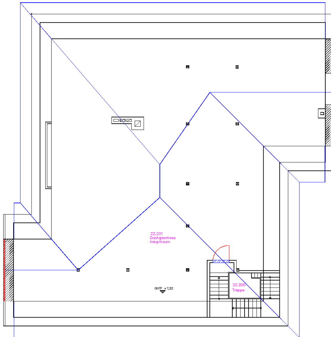
Abbildung 6: Grundriss - Dritte Etage
